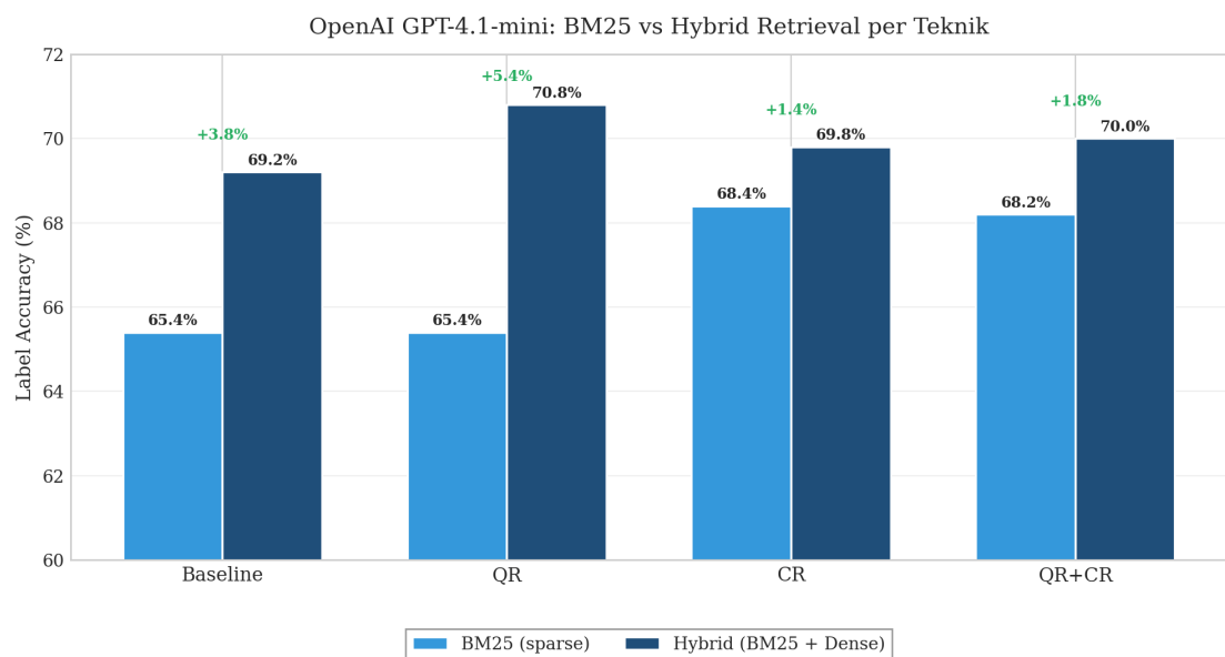
Gambar VI.1 Perbandingan akurasi label antara BM25 saja dengan Hybrid Retrieval pada GPT-4.1-mini
