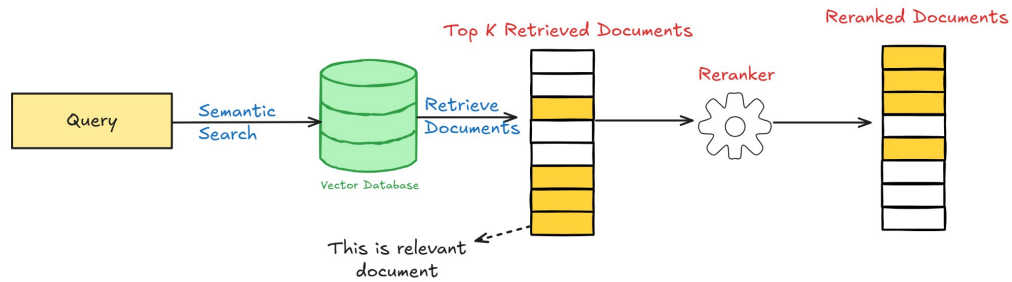
Gambar II.3 Alur kerja context reranking pada sistem RAG (Arooj March 2025)
